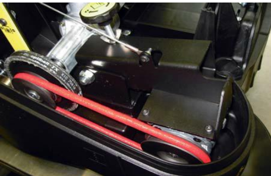
Bezkońcowe, elastyczne pasy okrągłe, czerwone PU, w przegrodzie silnikowej maszyny czyszczącej
