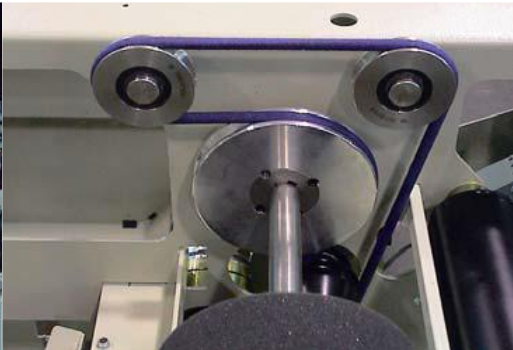
Napęd rolkowy w maszynie plecącej
