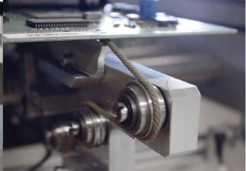
3,0 mm pas okrągły PBO podtrzymujący płytę z obwodami w maszynie lutującej przy temp. 380° C
