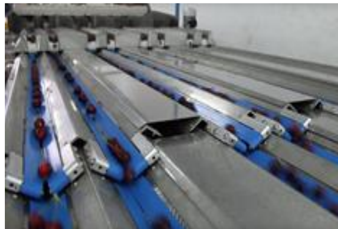
Längsgerillte Keilleistengurte beim Transport von Kirschen und Äpfeln von der Wascheinheit zur Größensortierung.
