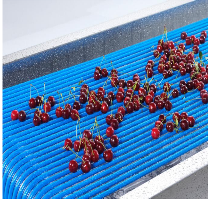
Wascheinheit mit Typ 820 75 Sh.A EU/FDA
