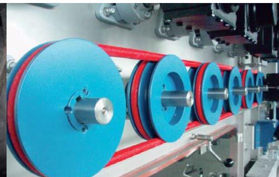
Oberwalzenantrieb in einem Efecta-Abteil einer Stoffwaschmaschine
