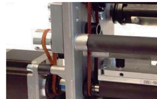
Vulkollan-Rundriemen in einem Etikettendruckwerk Gedrehte Rundriemen aus Kevlar in einer Transportstrecke für Abdeckrahmen
